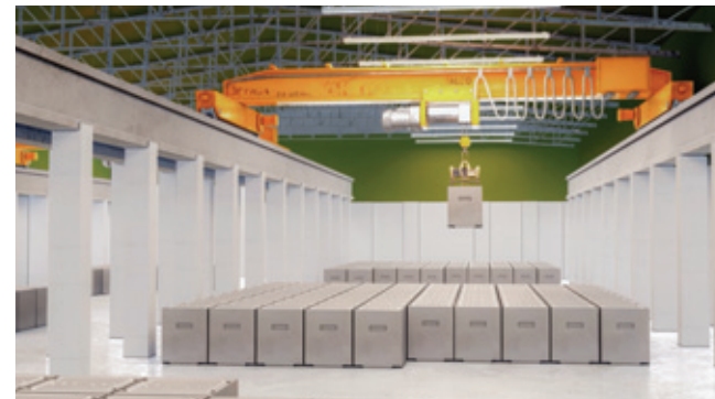
Unutrašnjost skladišta za NSRAO iz NE Krško
