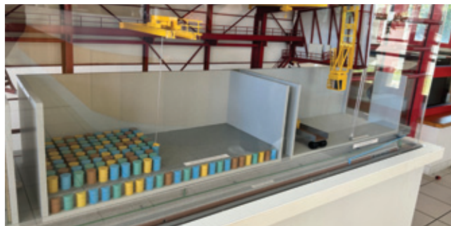
Maketa odlagališne jedinice u Info centru francuskog nacionalnog odlagališta
